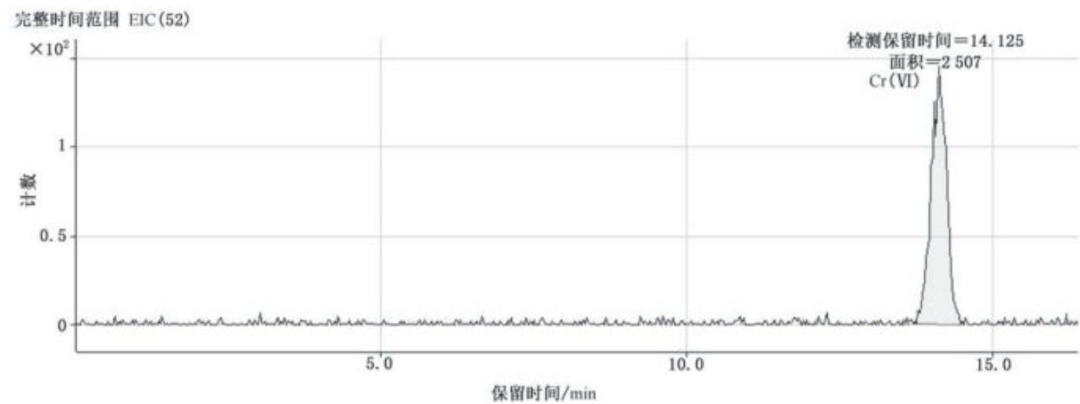
图 A.1 六价铬标准溶液谱图(质量数 52)
