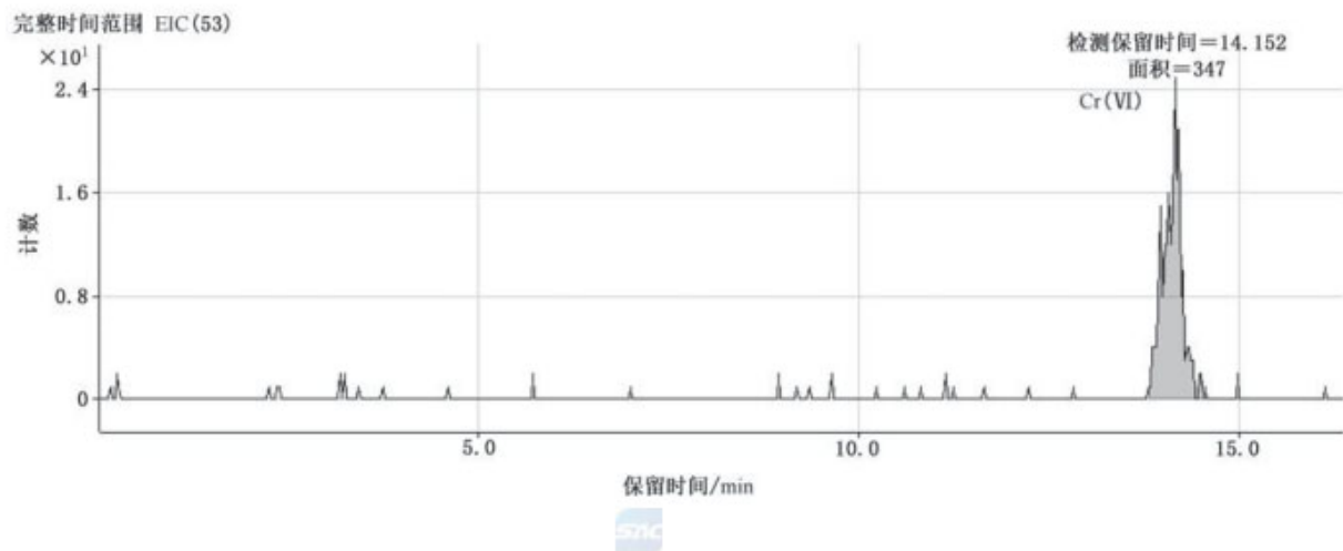
图 A.2 六价铬标准溶液谱图(质量数 53)
